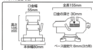
バイスの各部寸法
